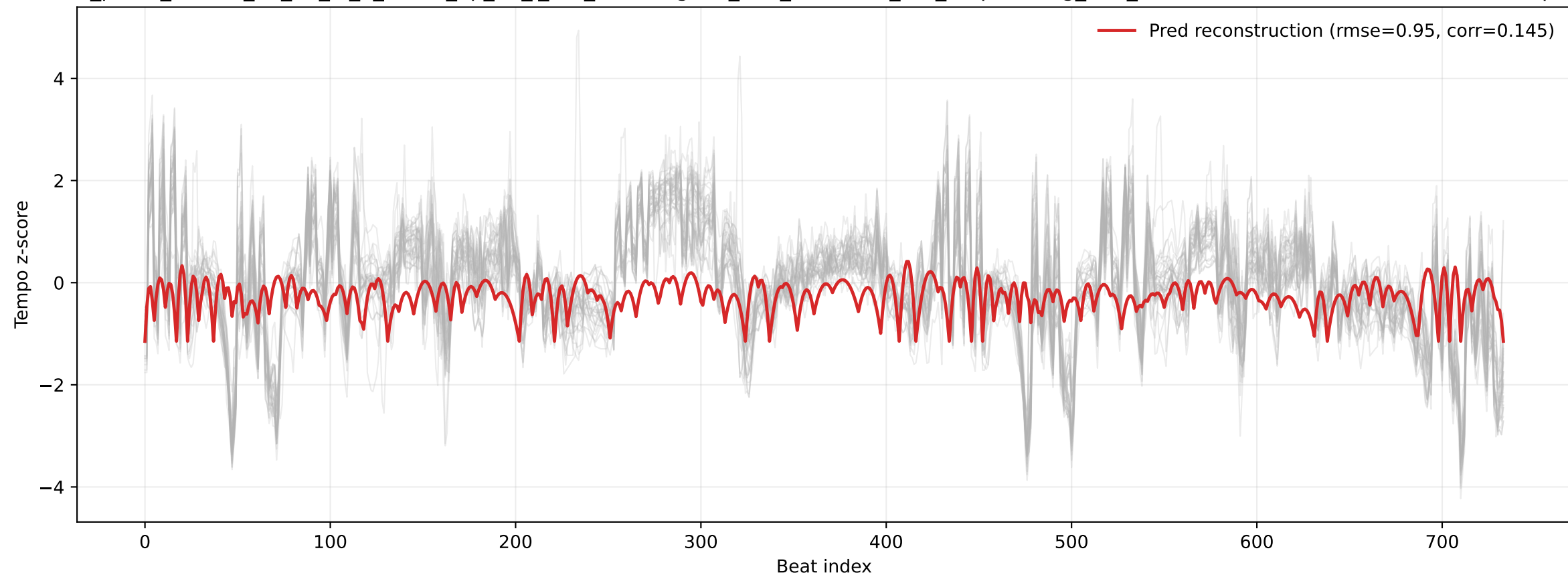
ludwig_van_beethoven_piano_sonata_no_27_in_e_minor_op_90_i_mit_lebhaftigkeit_und_durchaus_mit_empfindung_und_ausdruck: Pred reconstruction vs ALL performer tempo curves
